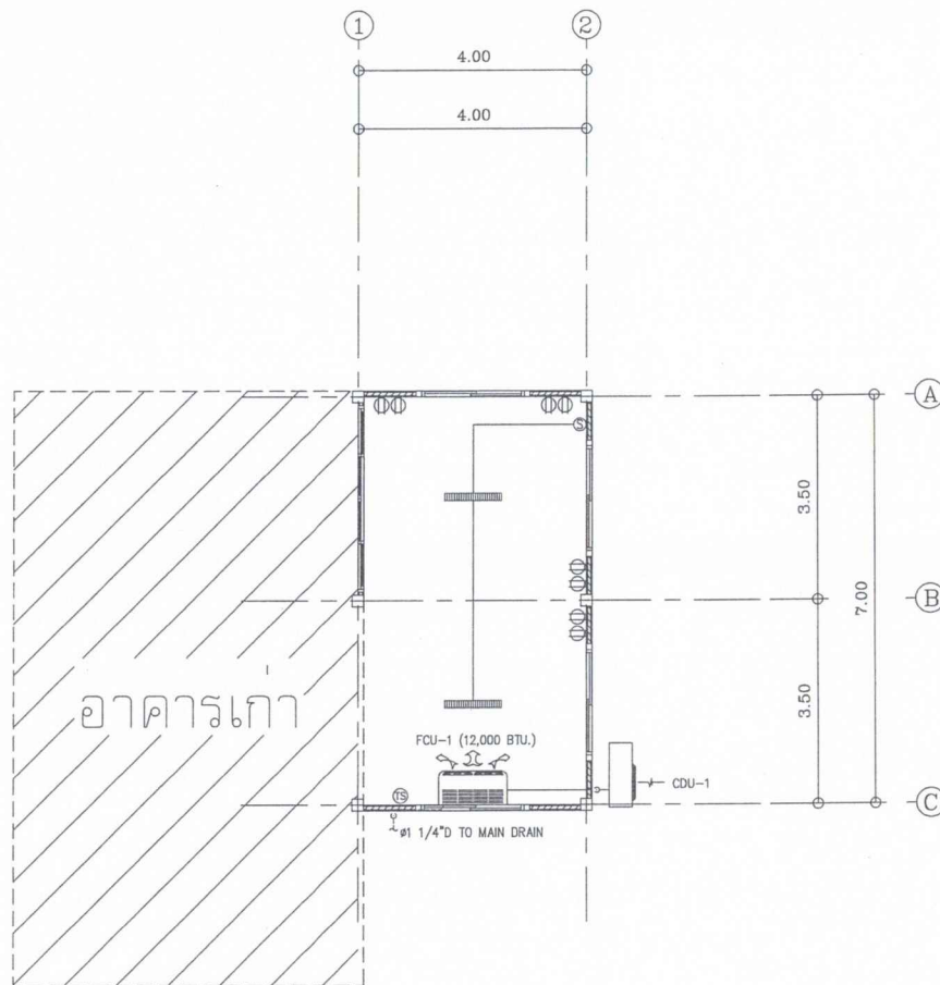
แปลนไฟฟ้า SCALE 1 : 100
