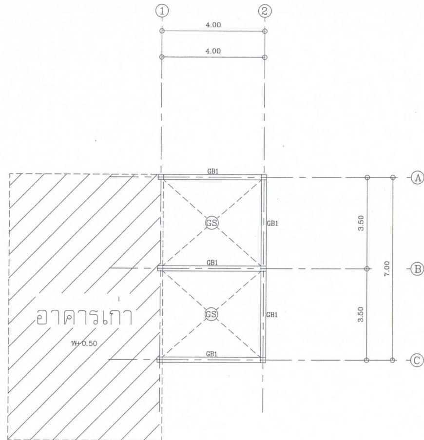
แปลนคาน พื้น SCALE 1 : 100
