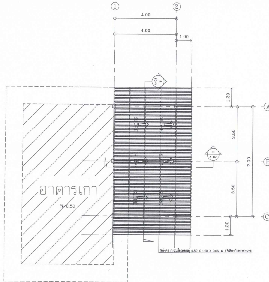
แปลนหลังคา SCALE 1 : 100
